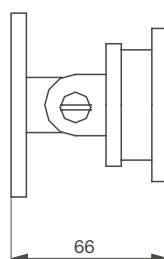
➤ Contreplaque fournie avec la ventouse V7E (réf. V7PM0110000)
