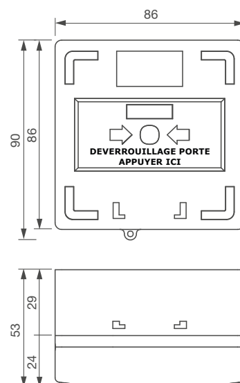
➤ RCP100BK
