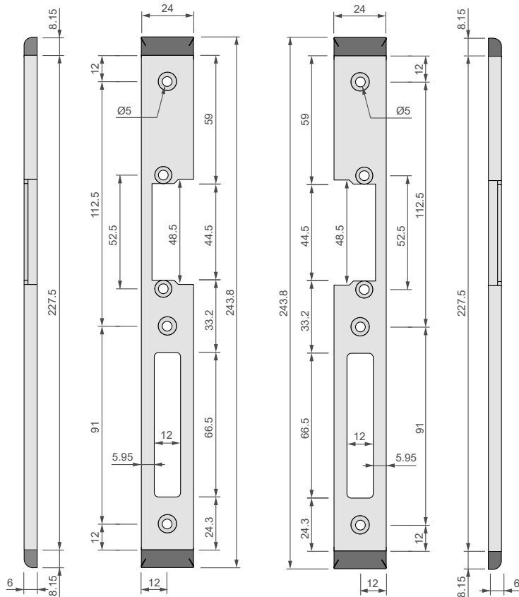
SP24424-E1SLX (DIN gauche)
