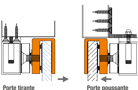
Porte tirante sous traverse
