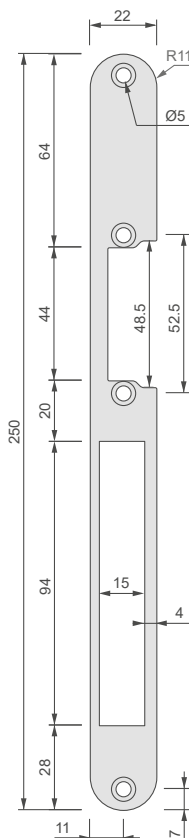
SP25022-F1RUX
