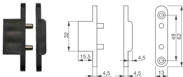
➤ PCT200
