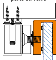
Porte tirante sous traverse
