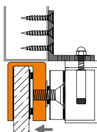
Porte poussante (à commander avec la référence EMS300L)
