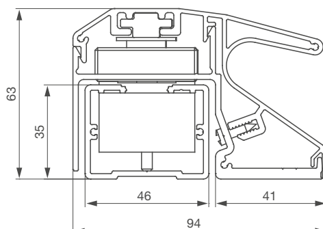
Coupe du profilé
