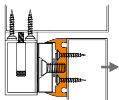
Porte tirante sous traverse
