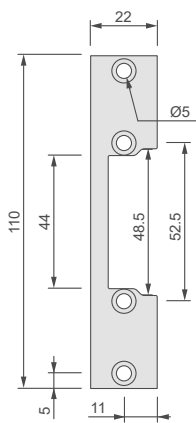
SP11022-Q1SUX
