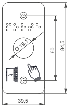
➤ SSP101
