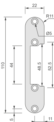
SP11022-Q1RUX
