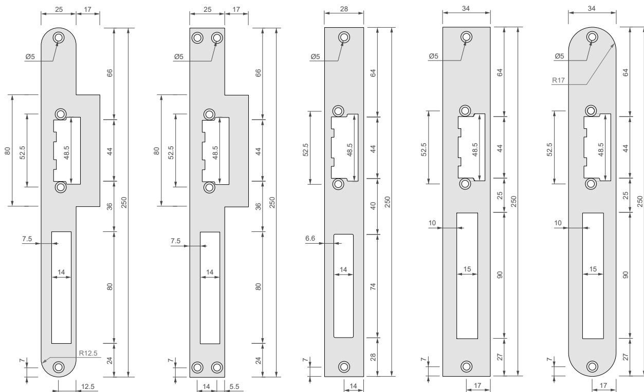
SP25025-L1RUX
