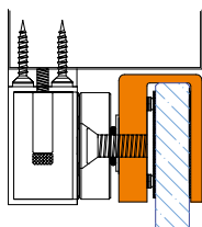
Porte tirante sous traverse
