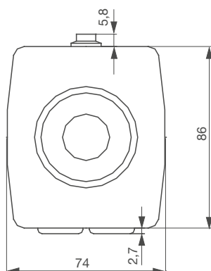
➤ Ventouse V7E
