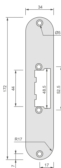
SP17234-V1RUX
