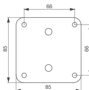
➤ Vue de côté applique
